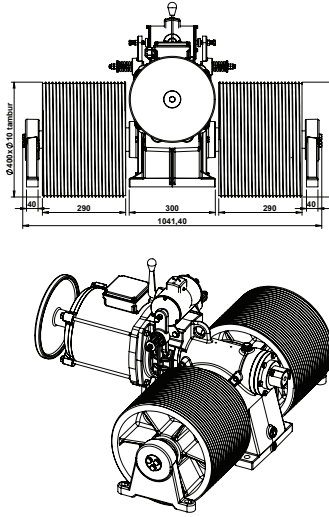
AKIS ZF 82-7,5 kW 26M. ÇİFT TAMBUR TEK HALAT
